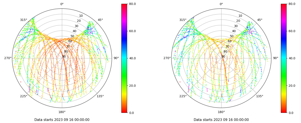
Skyplot for station LPAL. Parameter M1C Data file LPAL00ESP_R_2023259.xtr Skyplot for station LPAL. Parameter M2S Data file LPAL00ESP_R_2023259.xtr
