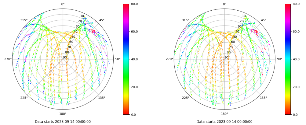
Skyplot for station LPAL. Parameter M1C Data file LPAL00ESP_R_2023257.xtr Skyplot for station LPAL. Parameter M2C Data file LPAL00ESP_R_2023257.xtr
