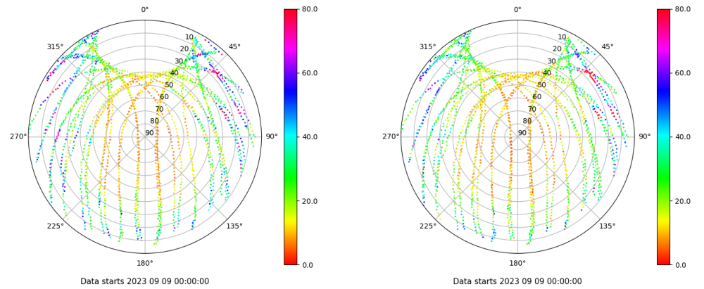
Skyplot for station LPAL. Parameter M1C Data file LPAL00ESP_R_2023252.xtr Skyplot for station LPAL. Parameter M2C Data file LPAL00ESP_R_2023252.xtr
