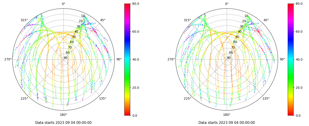
Skyplot for station LPAL. Parameter M1C Data file LPAL00ESP_R_2023247.xtr Skyplot for station LPAL. Parameter M2C Data file LPAL00ESP_R_2023247.xtr
