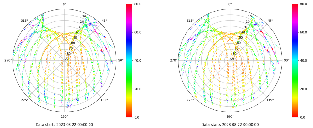
Skyplot for station LPAL. Parameter M1C Data file LPAL00ESP_R_2023234.xtr Skyplot for station LPAL. Parameter M2C Data file LPAL00ESP_R_2023234.xtr
