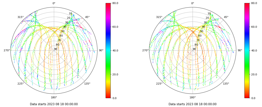
Skyplot for station LPAL. Parameter M1C Data file LPAL00ESP_R_2023230.xtr Skyplot for station LPAL. Parameter M2C Data file LPAL00ESP_R_2023230.xtr
