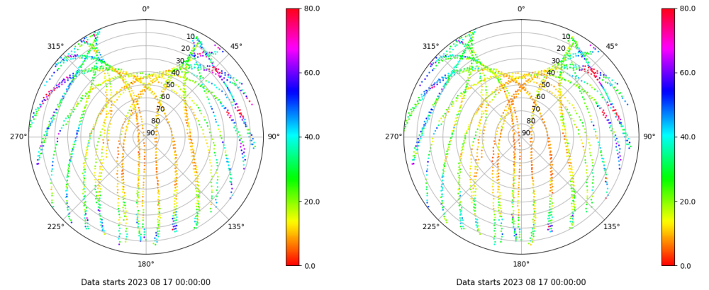
Skyplot for station LPAL. Parameter M1C Data file LPAL00ESP_R_2023229.xtr Skyplot for station LPAL. Parameter M2C Data file LPAL00ESP_R_2023229.xtr
