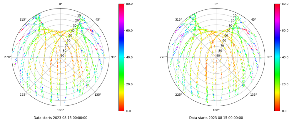
Skyplot for station LPAL. Parameter M1C Data file LPAL00ESP_R_2023227.xtr Skyplot for station LPAL. Parameter M2C Data file LPAL00ESP_R_2023227.xtr
