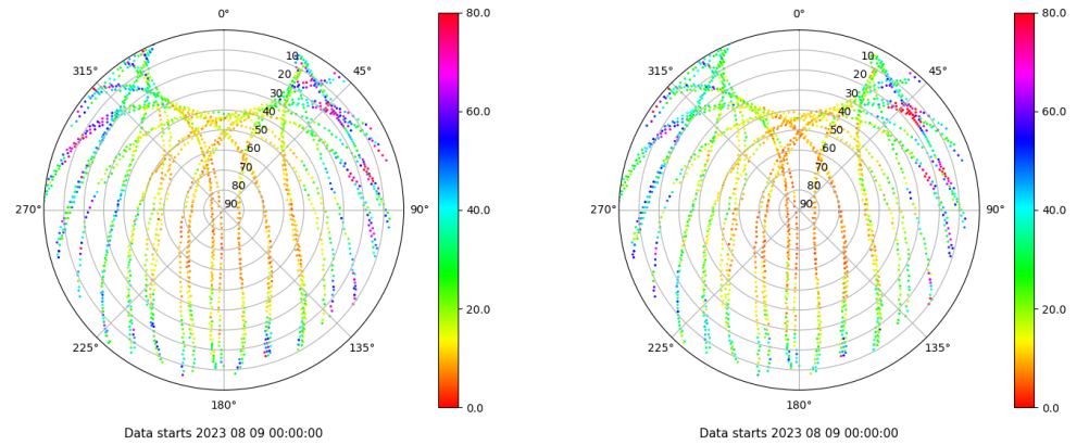
Skyplot for station LPAL. Parameter M1C Data file LPAL00ESP_R_2023221.xtr Skyplot for station LPAL. Parameter M2C Data file LPAL00ESP_R_2023221.xtr
