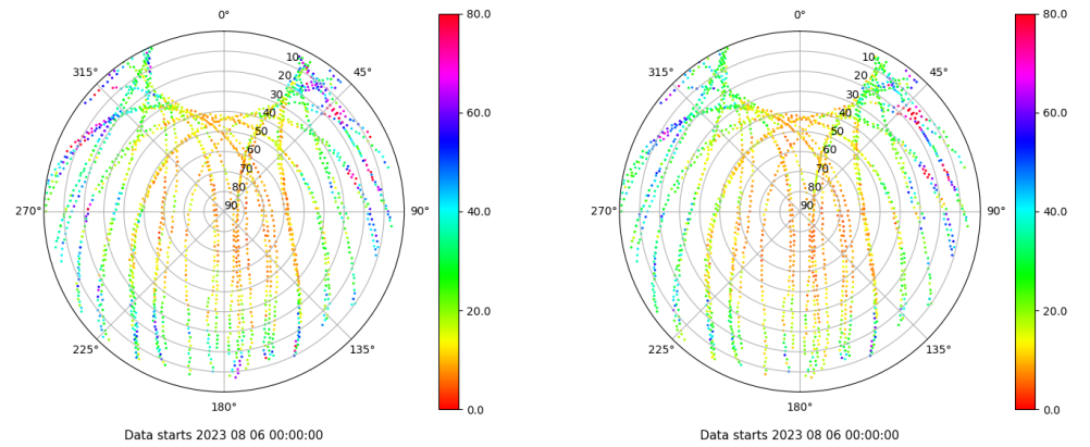
Skyplot for station LPAL. Parameter M1C Data file LPAL00ESP_R_2023218.xtr Skyplot for station LPAL. Parameter M2C Data file LPAL00ESP_R_2023218.xtr
