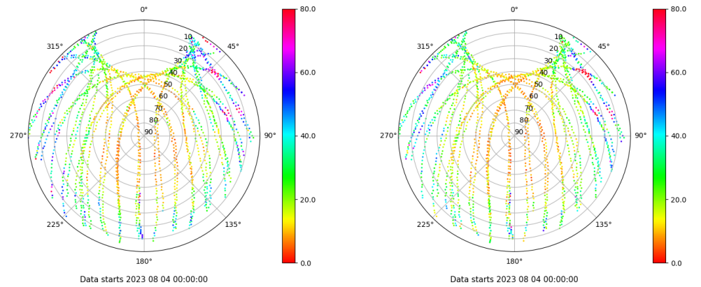
Skyplot for station LPAL. Parameter M1C Data file LPAL00ESP_R_2023216.xtr Skyplot for station LPAL. Parameter M2C Data file LPAL00ESP_R_2023216.xtr
