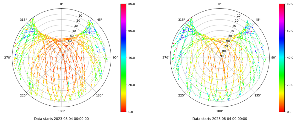
Skyplot for station LPAL. Parameter M1C Data file LPAL00ESP_R_2023216.xtr Skyplot for station LPAL. Parameter M2S Data file LPAL00ESP_R_2023216.xtr
