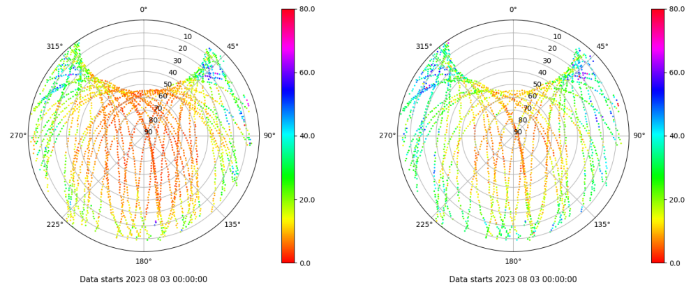
Skyplot for station LPAL. Parameter M1C Data file LPAL00ESP_R_2023215.xtr Skyplot for station LPAL. Parameter M2S Data file LPAL00ESP_R_2023215.xtr
