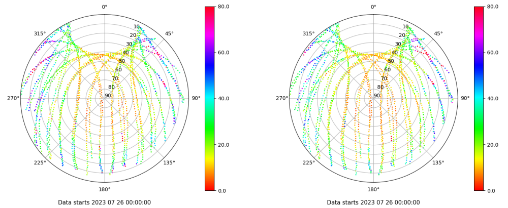
Skyplot for station LPAL. Parameter M1C Data file LPAL00ESP_R_2023207.xtr Skyplot for station LPAL. Parameter M2C Data file LPAL00ESP_R_2023207.xtr
