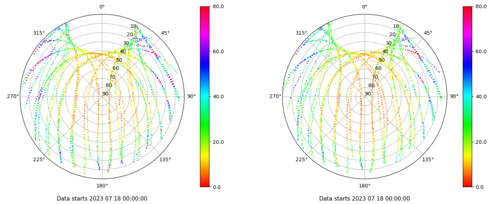
Skyplot for station LPAL. Parameter M1C Data file LPAL00ESP_R_2023199.xtr Skyplot for station LPAL. Parameter M2C Data file LPAL00ESP_R_2023199.xtr
