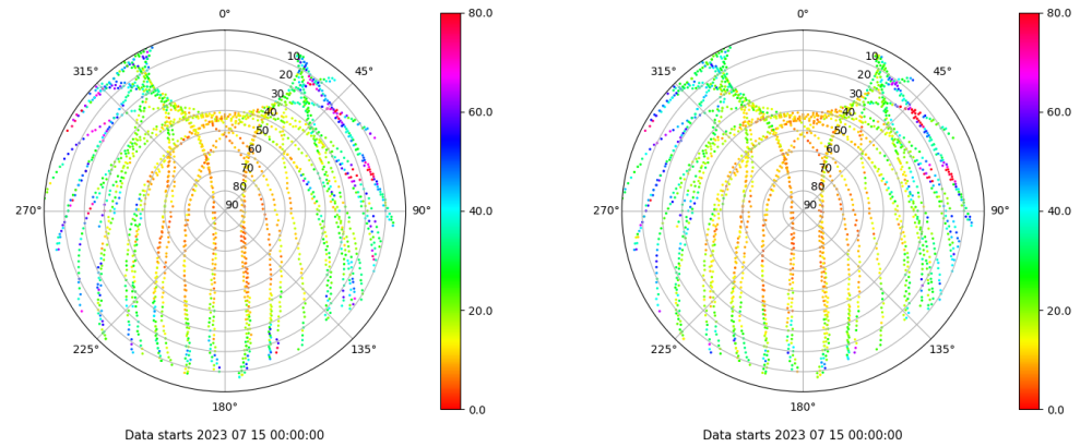
Skyplot for station LPAL. Parameter M1C Data file LPAL00ESP_R_2023196.xtr Skyplot for station LPAL. Parameter M2C Data file LPAL00ESP_R_2023196.xtr
