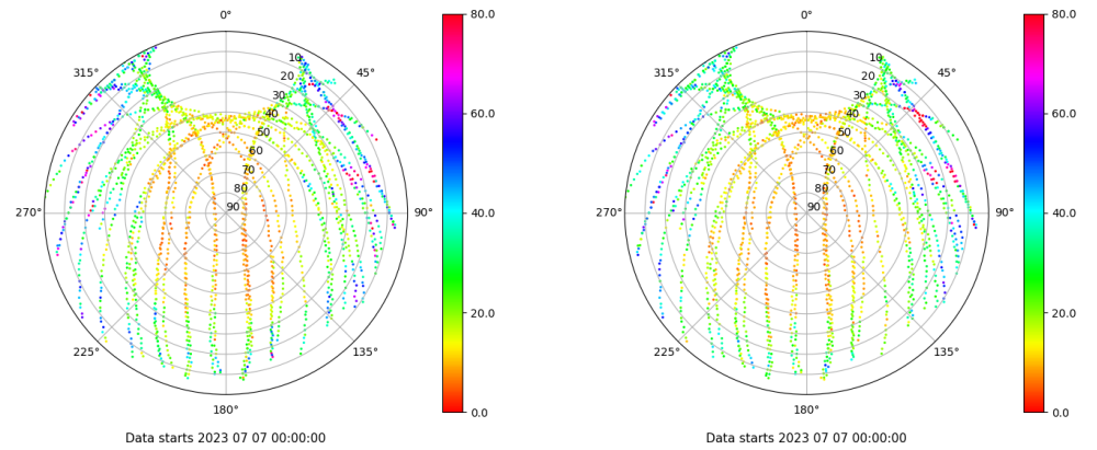
Skyplot for station LPAL. Parameter M1C Data file LPAL00ESP_R_2023188.xtr Skyplot for station LPAL. Parameter M2C Data file LPAL00ESP_R_2023188.xtr
