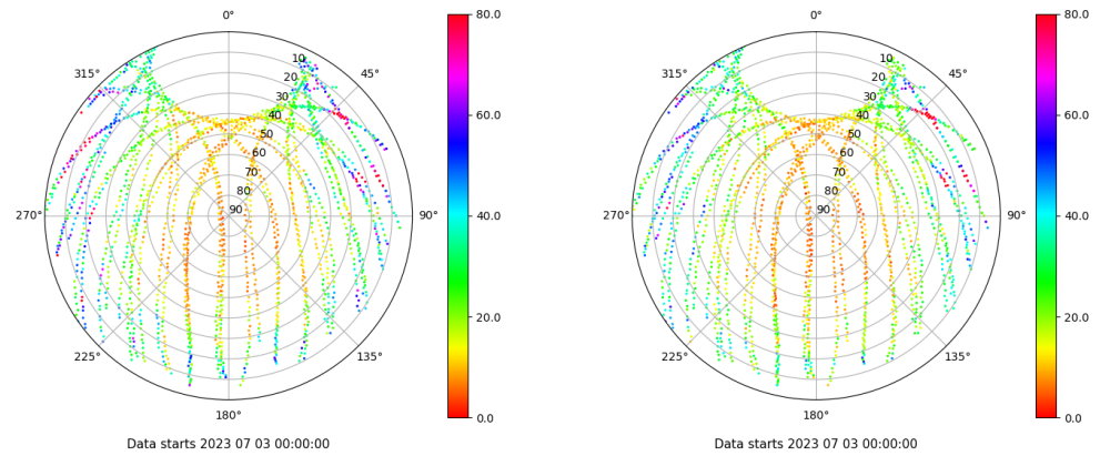
Skyplot for station LPAL. Parameter M1C Data file LPAL00ESP_R_2023184.xtr Skyplot for station LPAL. Parameter M2C Data file LPAL00ESP_R_2023184.xtr
