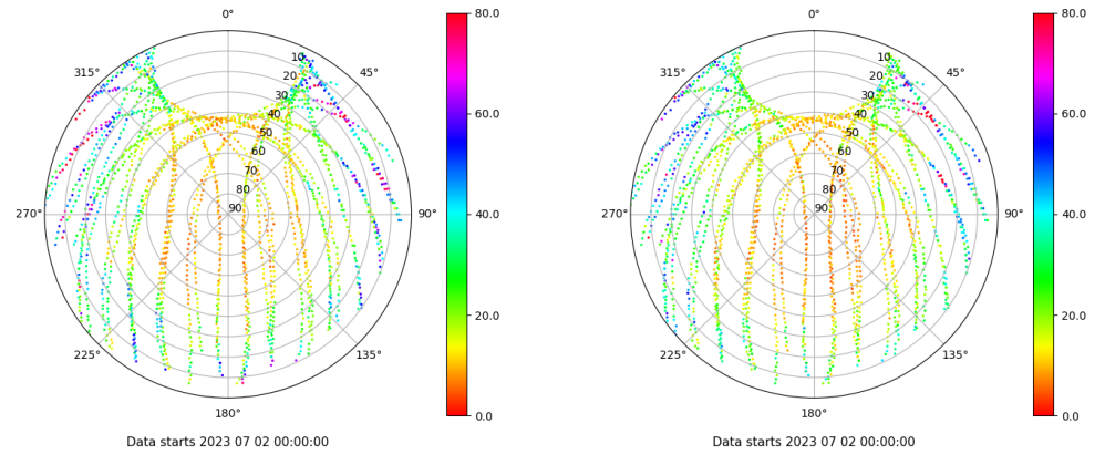
Skyplot for station LPAL. Parameter M1C Data file LPAL00ESP_R_2023183.xtr Skyplot for station LPAL. Parameter M2C Data file LPAL00ESP_R_2023183.xtr
