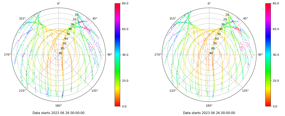
Skyplot for station LPAL. Parameter M1C Data file LPAL00ESP_R_2023177.xtr Skyplot for station LPAL. Parameter M2C Data file LPAL00ESP_R_2023177.xtr
