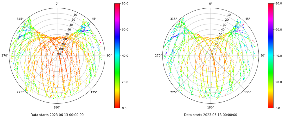
Skyplot for station LPAL. Parameter M1C Data file LPAL00ESP_R_2023164.xtr Skyplot for station LPAL. Parameter M2S Data file LPAL00ESP_R_2023164.xtr
