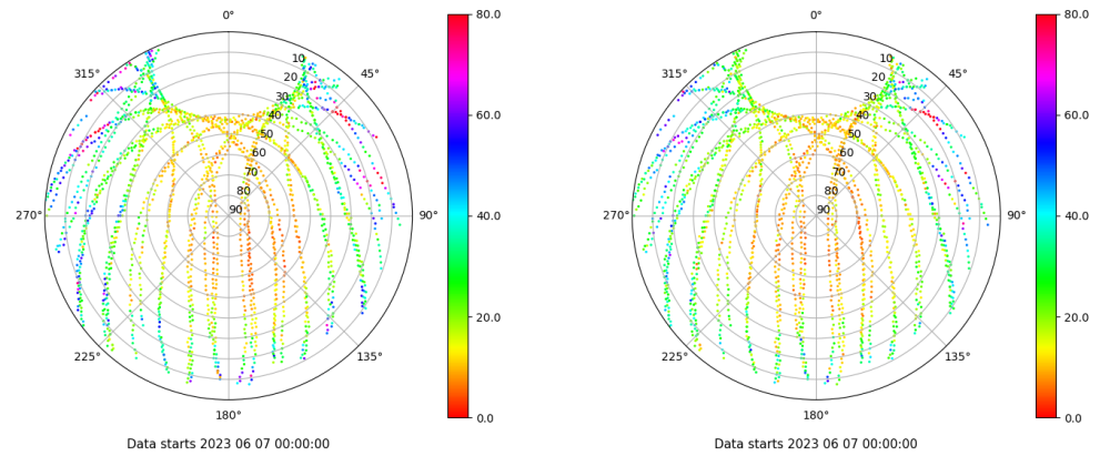
Skyplot for station LPAL. Parameter M1C Data file LPAL00ESP_R_2023158.xtr Skyplot for station LPAL. Parameter M2C Data file LPAL00ESP_R_2023158.xtr
