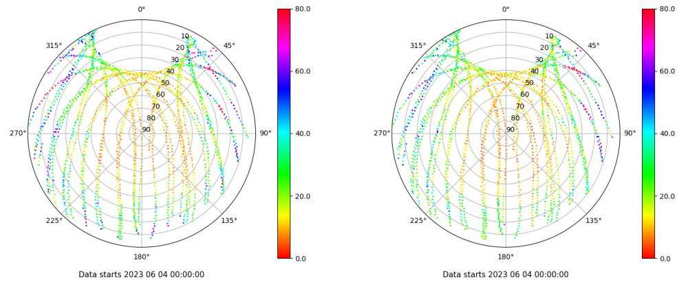
Skyplot for station LPAL. Parameter M1C Data file LPAL00ESP_R_2023155.xtr Skyplot for station LPAL. Parameter M2C Data file LPAL00ESP_R_2023155.xtr
