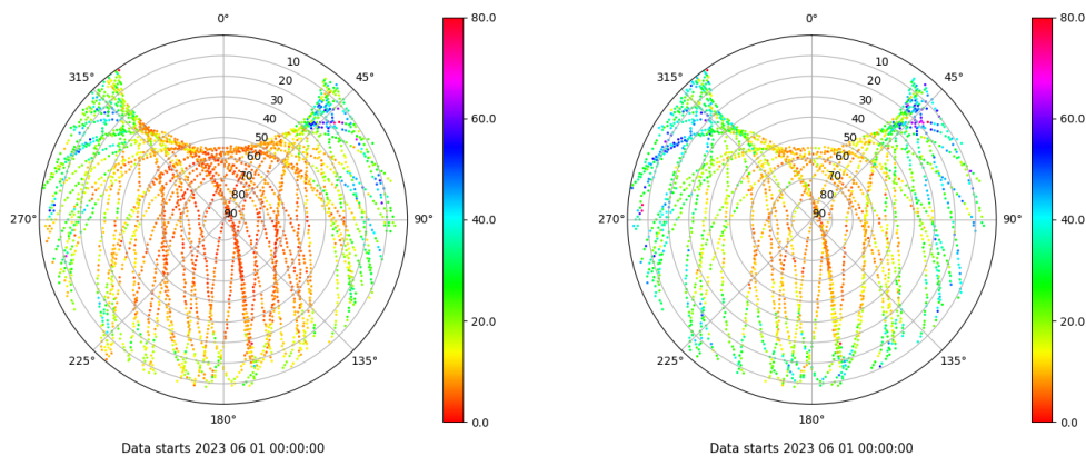
Skyplot for station LPAL. Parameter M1C Data file LPAL00ESP_R_2023152.xtr Skyplot for station LPAL. Parameter M2S Data file LPAL00ESP_R_2023152.xtr
