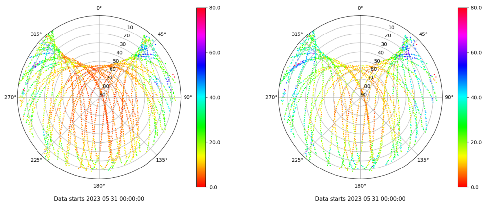
Skyplot for station LPAL. Parameter M1C Data file LPAL00ESP_R_2023151.xtr Skyplot for station LPAL. Parameter M2S Data file LPAL00ESP_R_2023151.xtr
