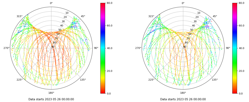
Skyplot for station LPAL. Parameter M1C Data file LPAL00ESP_R_2023146.xtr Skyplot for station LPAL. Parameter M2S Data file LPAL00ESP_R_2023146.xtr
