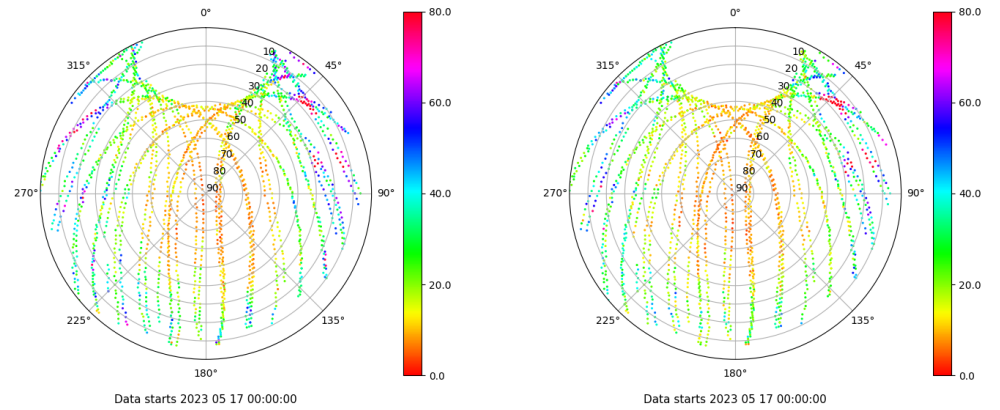
Skyplot for station LPAL. Parameter M1C Data file LPAL00ESP_R_2023137.xtr Skyplot for station LPAL. Parameter M2C Data file LPAL00ESP_R_2023137.xtr
