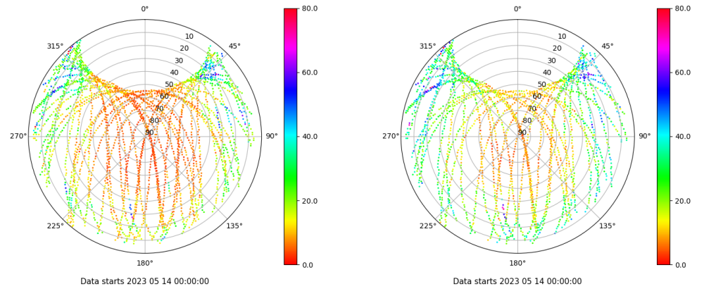
Skyplot for station LPAL. Parameter M1C Data file LPAL00ESP_R_2023134.xtr Skyplot for station LPAL. Parameter M2S Data file LPAL00ESP_R_2023134.xtr
