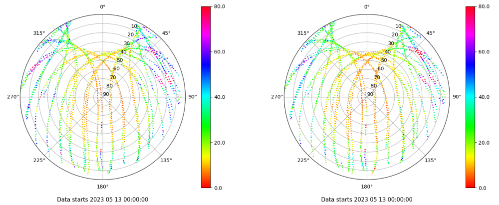
Skyplot for station LPAL. Parameter M1C Data file LPAL00ESP_R_2023133.xtr Skyplot for station LPAL. Parameter M2C Data file LPAL00ESP_R_2023133.xtr
