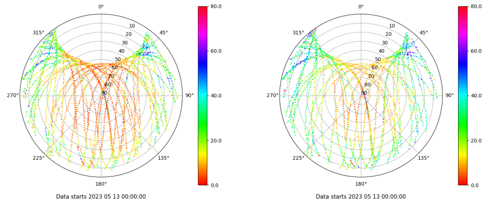
Skyplot for station LPAL. Parameter M1C Data file LPAL00ESP_R_2023133.xtr Skyplot for station LPAL. Parameter M2S Data file LPAL00ESP_R_2023133.xtr
