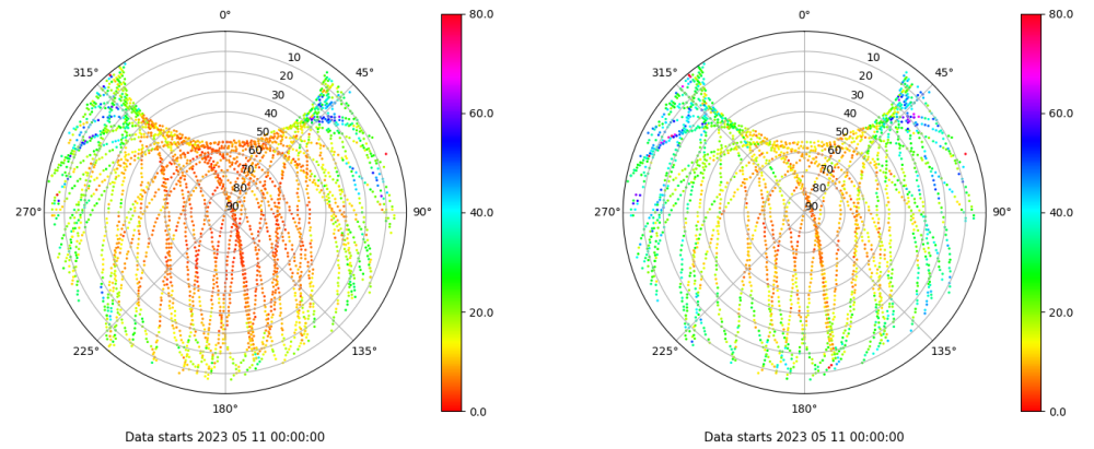
Skyplot for station LPAL. Parameter M1C Data file LPAL00ESP_R_2023131.xtr Skyplot for station LPAL. Parameter M2S Data file LPAL00ESP_R_2023131.xtr
