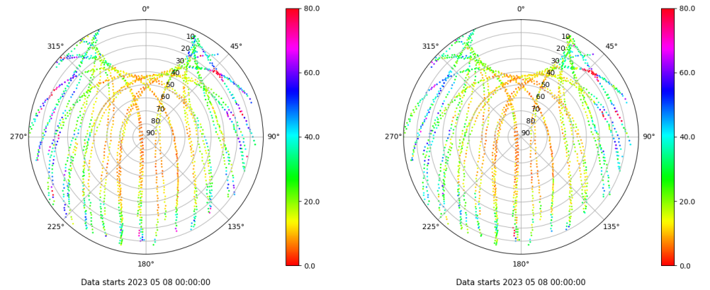
Skyplot for station LPAL. Parameter M1C Data file LPAL00ESP_R_2023128.xtr Skyplot for station LPAL. Parameter M2C Data file LPAL00ESP_R_2023128.xtr
