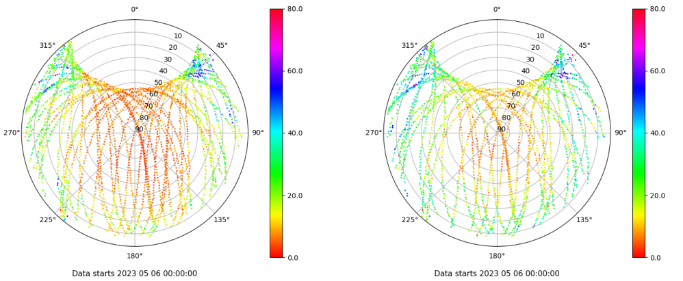
Skyplot for station LPAL. Parameter M1C Data file LPAL00ESP_R_2023126.xtr Skyplot for station LPAL. Parameter M2S Data file LPAL00ESP_R_2023126.xtr
