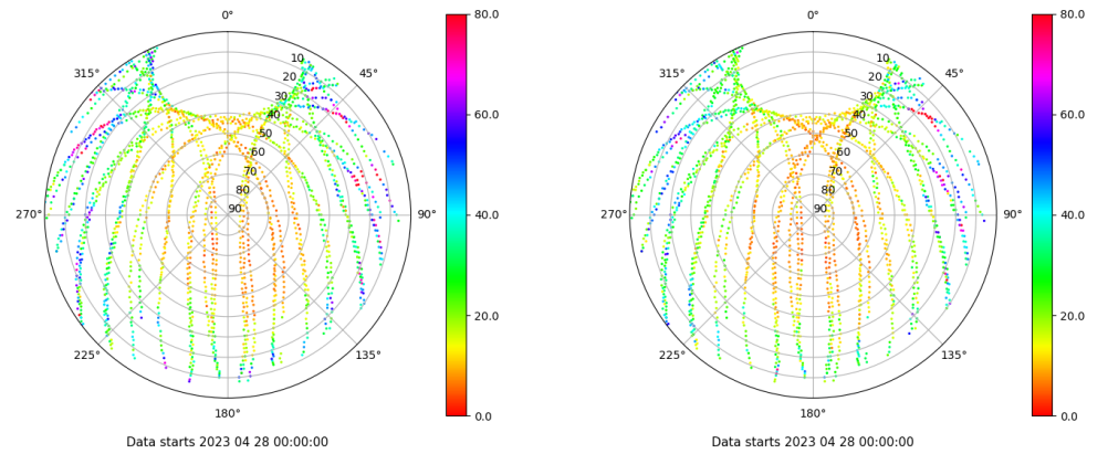
Skyplot for station LPAL. Parameter M1C Data file LPAL00ESP_R_2023118.xtr Skyplot for station LPAL. Parameter M2C Data file LPAL00ESP_R_2023118.xtr
