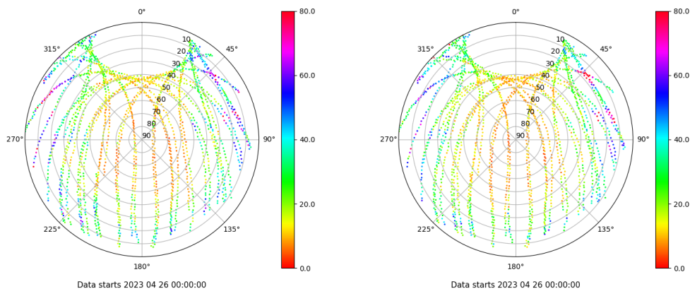
Skyplot for station LPAL. Parameter M1C Data file LPAL00ESP_R_2023116.xtr Skyplot for station LPAL. Parameter M2C Data file LPAL00ESP_R_2023116.xtr
