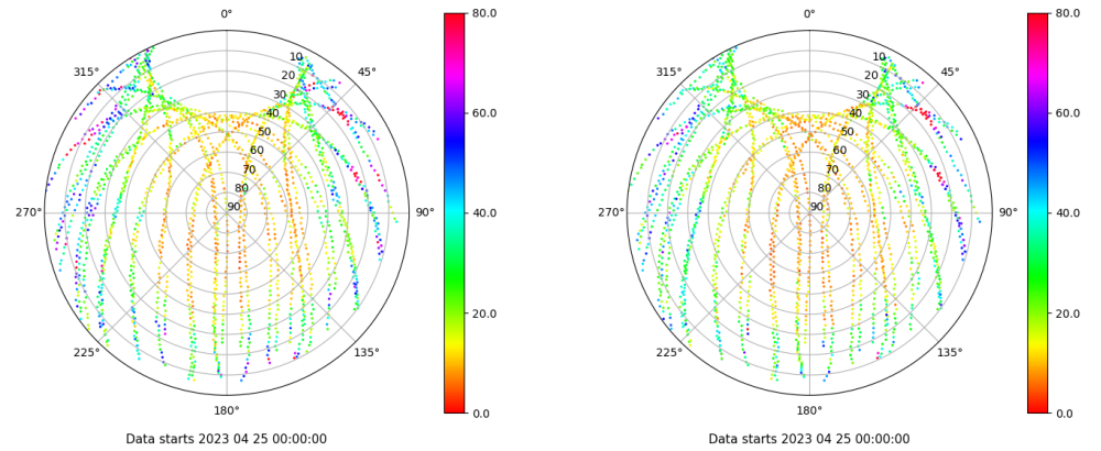
Skyplot for station LPAL. Parameter M1C Data file LPAL00ESP_R_2023115.xtr Skyplot for station LPAL. Parameter M2C Data file LPAL00ESP_R_2023115.xtr
