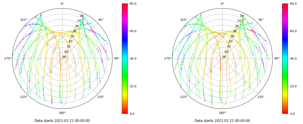
Skyplot for station LPAL. Parameter M1C Data file LPAL00ESP_R_2023080.xtr Skyplot for station LPAL. Parameter M2C Data file LPAL00ESP_R_2023080.xtr
