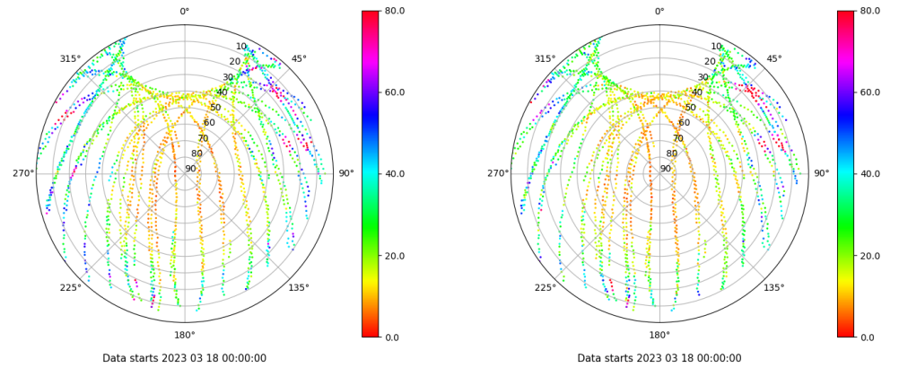
Skyplot for station LPAL. Parameter M1C Data file LPAL00ESP_R_2023077.xtr Skyplot for station LPAL. Parameter M2C Data file LPAL00ESP_R_2023077.xtr
