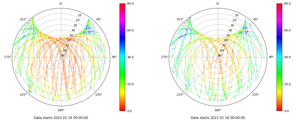
Skyplot for station LPAL. Parameter M1C Data file LPAL00ESP_R_2023016.xtr Skyplot for station LPAL. Parameter M2S Data file LPAL00ESP_R_2023016.xtr
