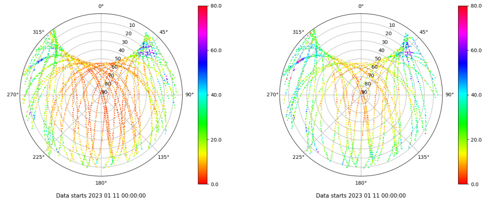
Skyplot for station LPAL. Parameter M1C Data file LPAL00ESP_R_2023011.xtr Skyplot for station LPAL. Parameter M2S Data file LPAL00ESP_R_2023011.xtr
