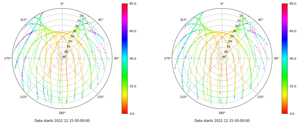
Skyplot for station LPAL. Parameter M1C Data file LPAL00ESP_R_2022359.xtr Skyplot for station LPAL. Parameter M2C Data file LPAL00ESP_R_2022359.xtr
