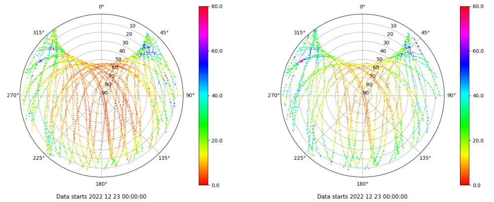
Skyplot for station LPAL. Parameter M1C Data file LPAL00ESP_R_2022357.xtr Skyplot for station LPAL. Parameter M2S Data file LPAL00ESP_R_2022357.xtr
