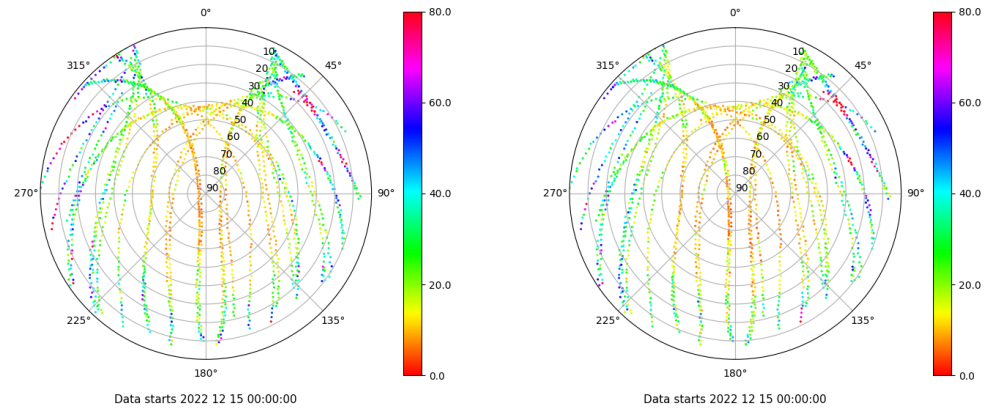
Skyplot for station LPAL. Parameter M1C Data file LPAL00ESP_R_2022349.xtr Skyplot for station LPAL. Parameter M2C Data file LPAL00ESP_R_2022349.xtr
