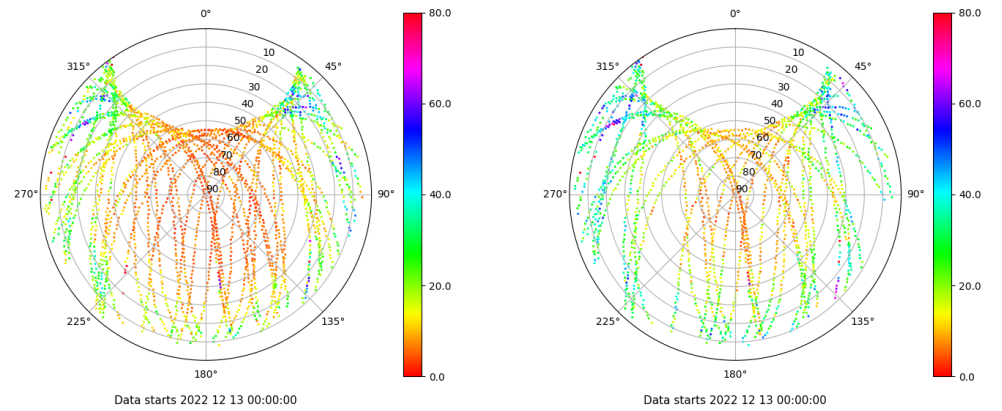
Skyplot for station LPAL. Parameter M1C Data file LPAL00ESP_R_2022347.xtr Skyplot for station LPAL. Parameter M2S Data file LPAL00ESP_R_2022347.xtr
