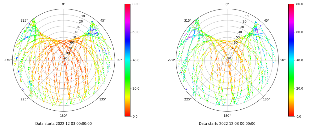
Skyplot for station LPAL. Parameter M1C Data file LPAL00ESP_R_2022337.xtr Skyplot for station LPAL. Parameter M2S Data file LPAL00ESP_R_2022337.xtr
