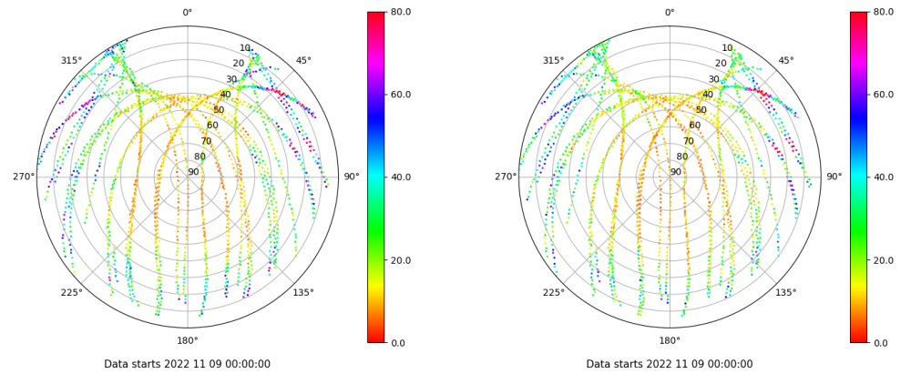
Skyplot for station LPAL. Parameter M1C Data file LPAL00ESP_R_2022313.xtr Skyplot for station LPAL. Parameter M2C Data file LPAL00ESP_R_2022313.xtr
