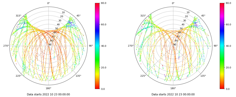
Skyplot for station LPAL. Parameter M1C Data file LPAL00ESP_R_2022296.xtr Skyplot for station LPAL. Parameter M2S Data file LPAL00ESP_R_2022296.xtr
