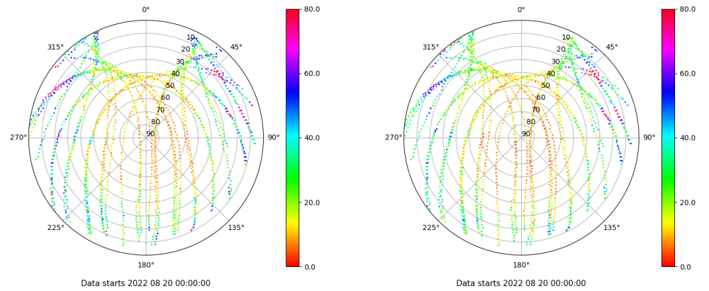
Skyplot for station LPAL. Parameter M1C Data file LPAL00ESP_R_2022232.xtr Skyplot for station LPAL. Parameter M2C Data file LPAL00ESP_R_2022232.xtr
