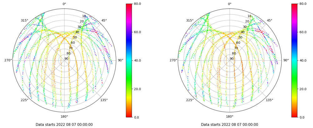
Skyplot for station LPAL. Parameter M1C Data file LPAL00ESP_R_2022219.xtr Skyplot for station LPAL. Parameter M2C Data file LPAL00ESP_R_2022219.xtr
