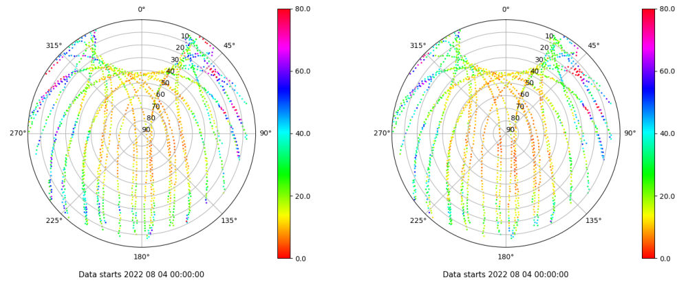
Skyplot for station LPAL. Parameter M1C Data file LPAL00ESP_R_2022216.xtr Skyplot for station LPAL. Parameter M2C Data file LPAL00ESP_R_2022216.xtr
