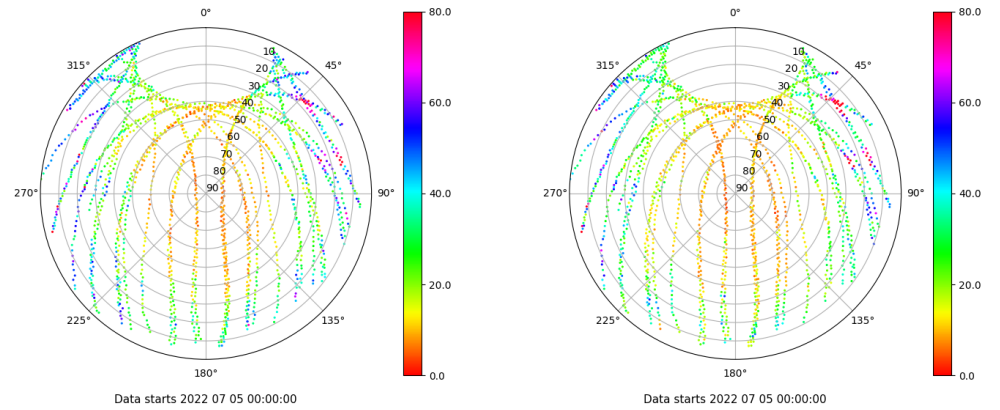
Skyplot for station LPAL. Parameter M1C Data file LPAL00ESP_R_2022186.xtr Skyplot for station LPAL. Parameter M2C Data file LPAL00ESP_R_2022186.xtr
