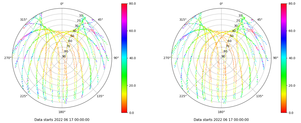
Skyplot for station LPAL. Parameter M1C Data file LPAL00ESP_R_2022168.xtr Skyplot for station LPAL. Parameter M2C Data file LPAL00ESP_R_2022168.xtr
